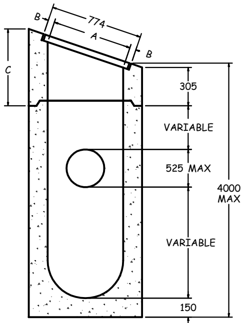
SECTION A-A 1:30
