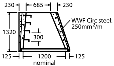
SECTION A-A TAPER CONE
