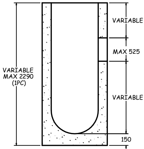
SECTION A-A 1:30
