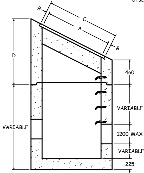
SECTION A-A 1:40
